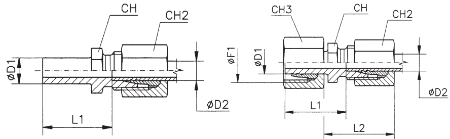
TN 132 Non serrato Sans écrou ni bague Not pre-assembled Unmontiert
