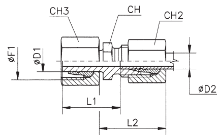
TN 132 A Serrato Avec écrou et bague présertis Pre-assembled Vormontiert
