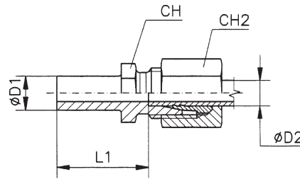
TN 132 Non serrato Sans écrou ni bague Not pre-assembled Unmontiert
